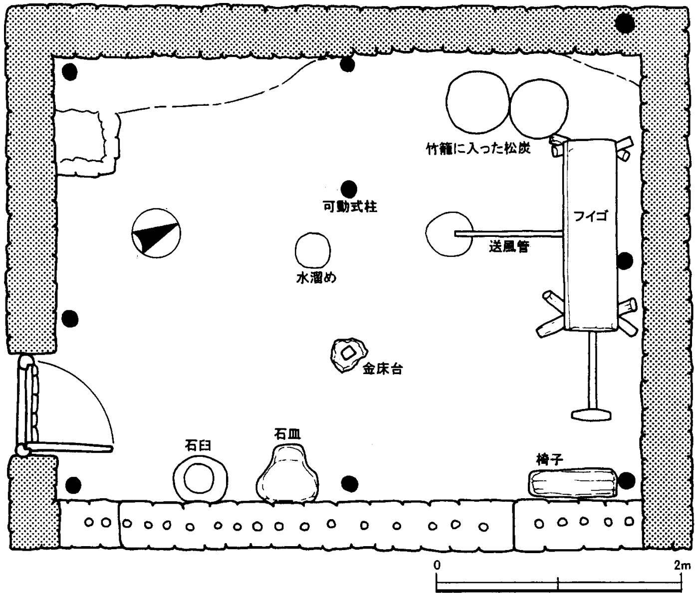
図3 俄垂大村の工房(1/50)
