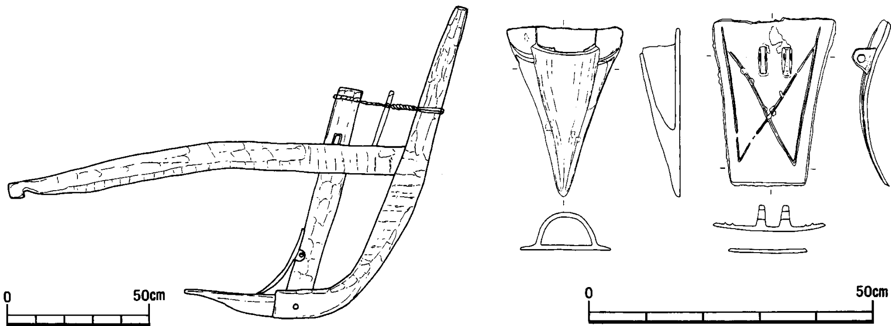
図2 牛犁(1/20)と犁先・撥土板(1/10)
