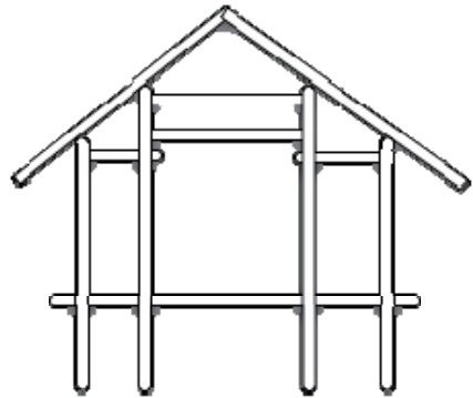
図5 フォン・トン・キーの構法
